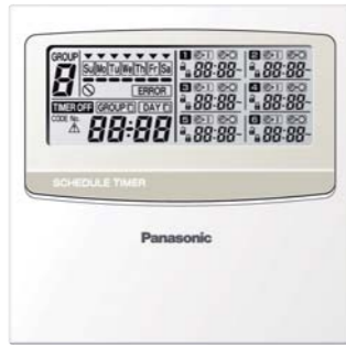
Габаритные размеры: (В x Ш x Г) 120 x 120 x 16 мм
